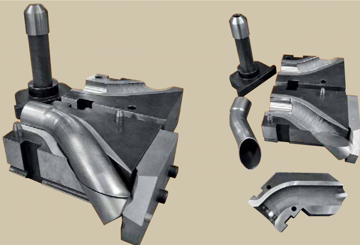
Cunas para el ensanchado en extremos de tubo
